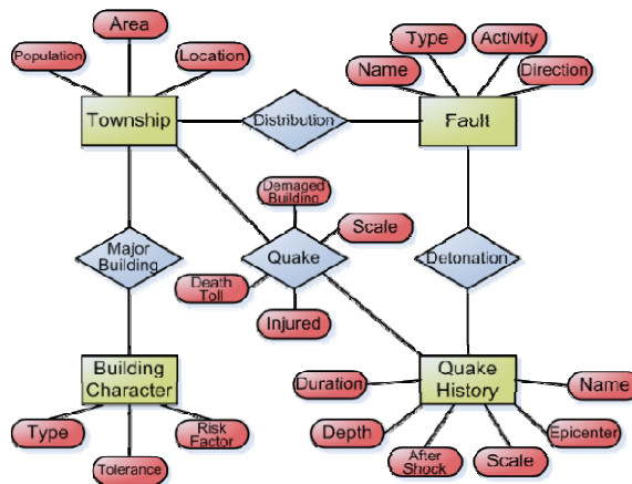
Fig. 2 ER Diagram of RISED
