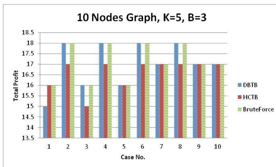
圖 38 實驗 1(a)：總效益比較
