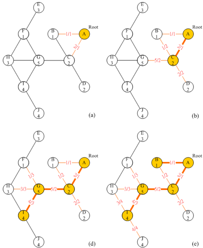
圖 37 HCTB 演算法步驟
