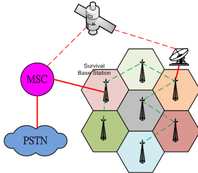
圖 12 CCN 網路示意圖
