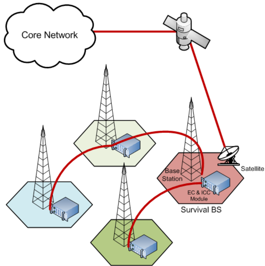
圖 17 CCN 通訊模式示意圖
