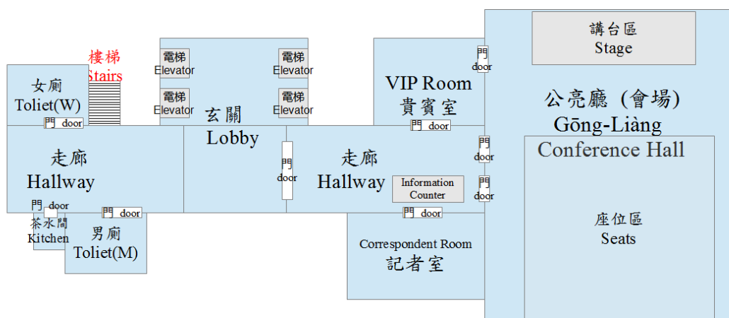
2F 公亮廳平面圖： The Second Floor plan:
